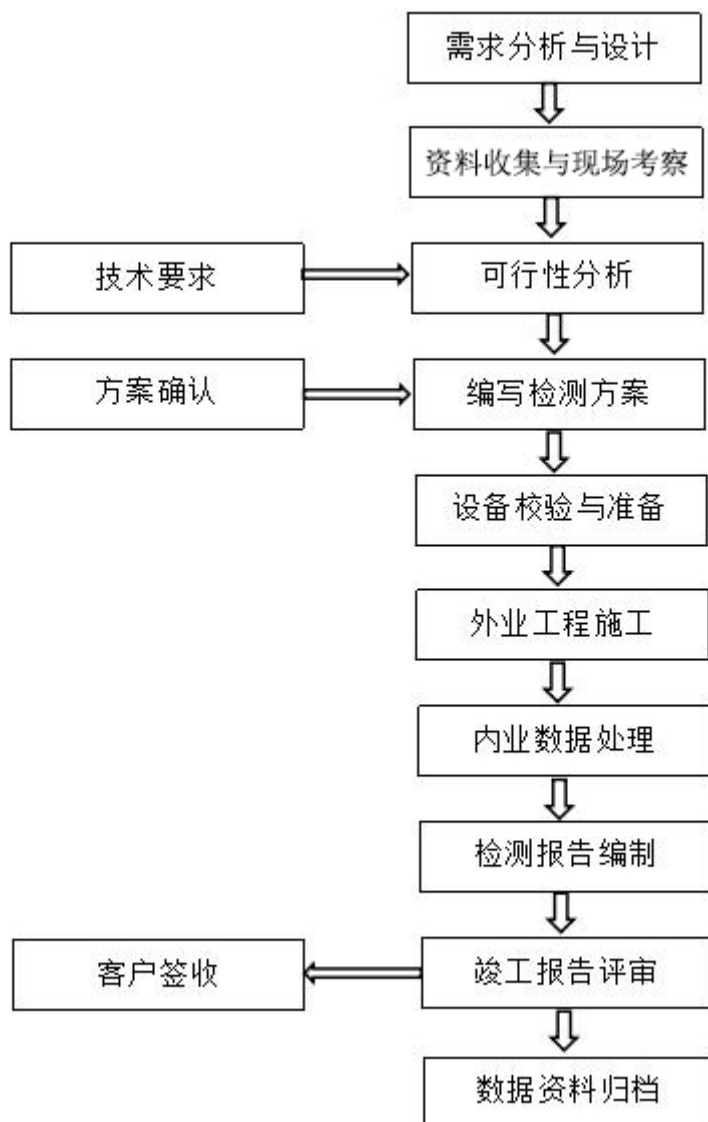
图 4.1 桥梁水下构件检测工作流程框图
